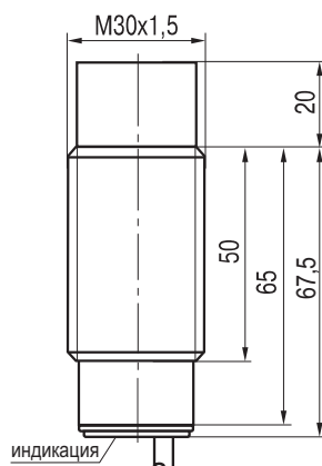
Габаритный чертеж
